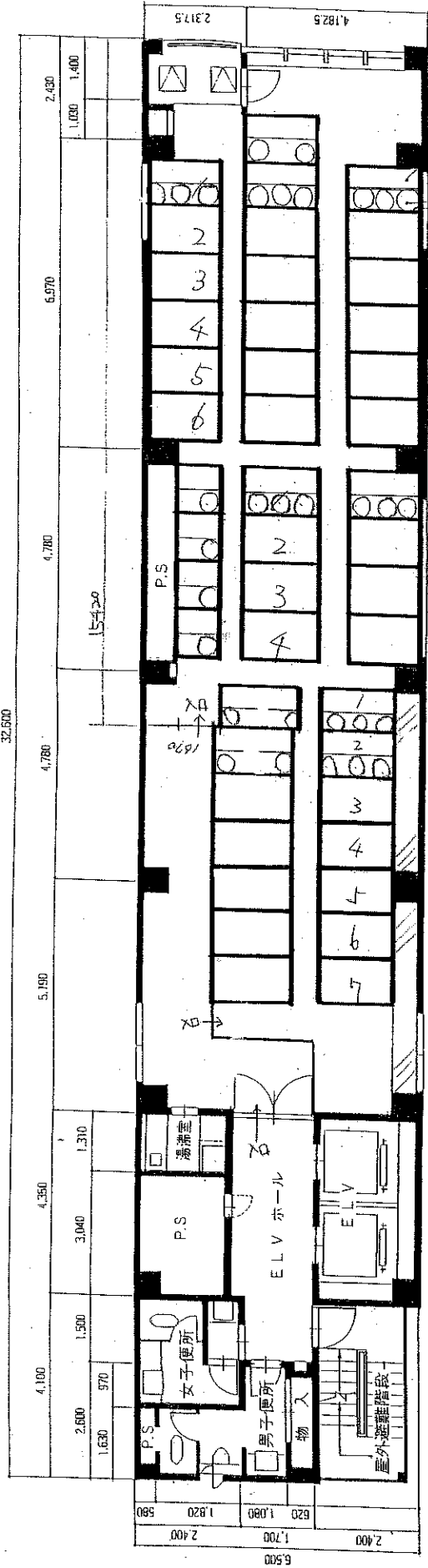
図六 平面
